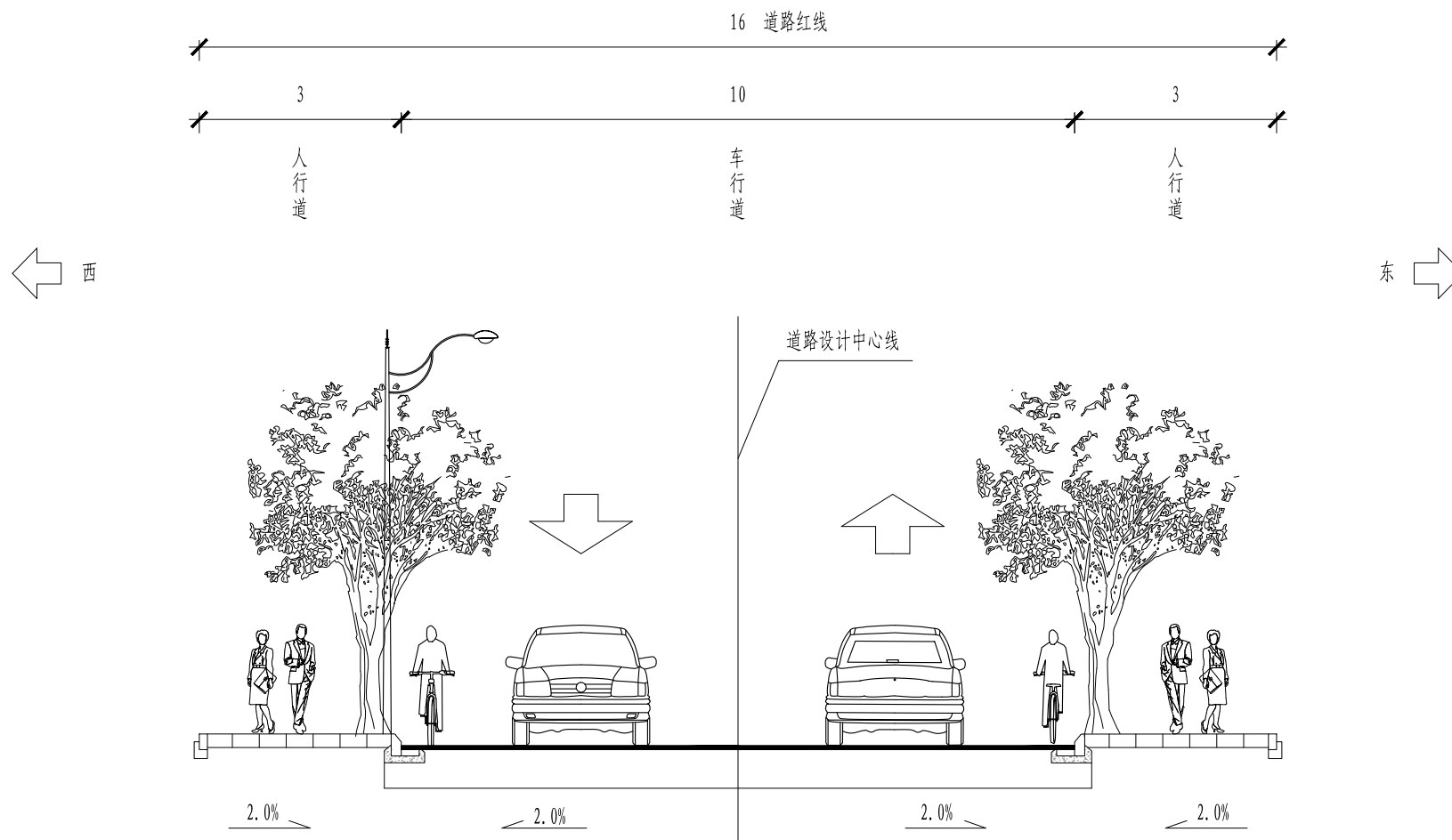
标准段横断面 推荐方案 1:100
